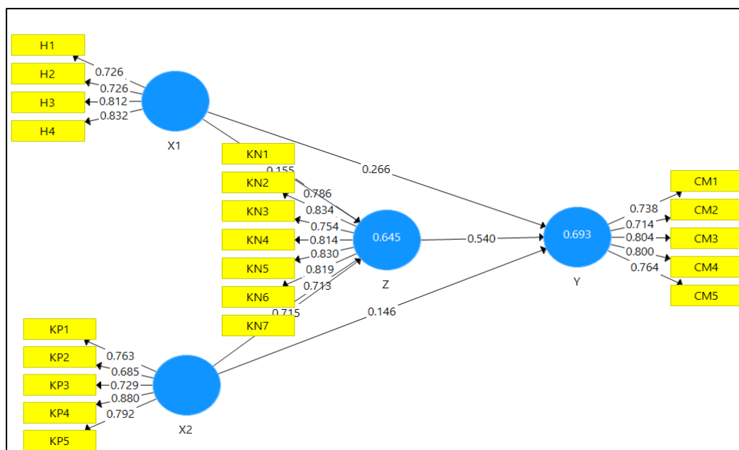
Gambar 1 Model Analisis Persamaan Struktural, Konstruk
